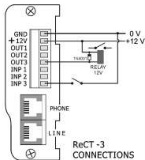
Σχήμα 1: Συνδέσεις του ReCT-3S
